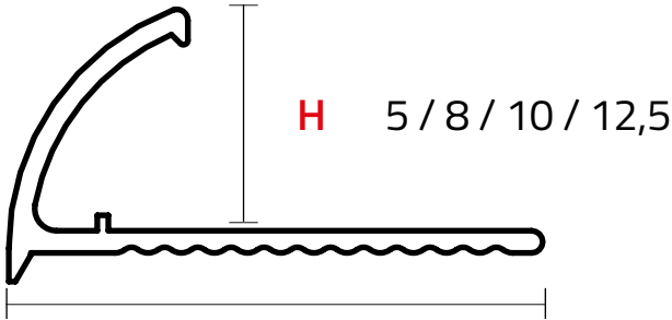
Protezione spigolo/ Corner protection
