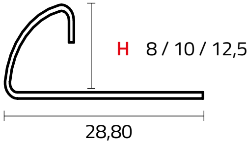
Protezione spigolo/ Corner protection
