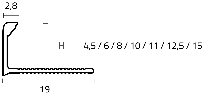
Chiusura perimetrale a pavimento/ Ground covering edging
