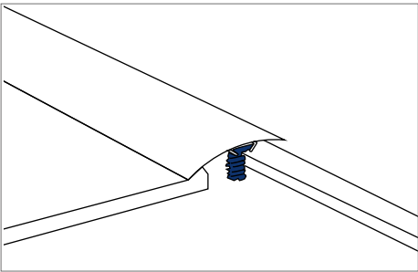
Sistema di montaggio con viti nascoste, incluse nell'articolo Installation system with hidden screws (included) Système de montage avec vis cachées, inclus dans l'article Sistema de montaje con tornillos ocultos, incluido en el artículo
