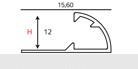
SOTTOPOSA - UNDERTILE
