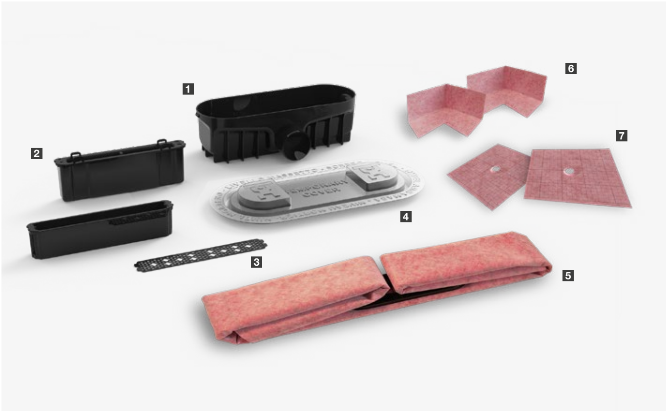
1- Scarico a scelta (TRYPHON, TRYPHON RIDOTTO o TRYPHON VERTICALE). 2- Sifone intercambiabile (idraulico e meccanico). 3- Raccogliacapelli. 4- Coperchio di livellamento del cemento. 5- Guaina WATER-STOP con connettore termosaldato. 6- W-S DIN x2 (rinforzo angolare interno). 7- W-S TUB x2 (tasello di tenuta ).
