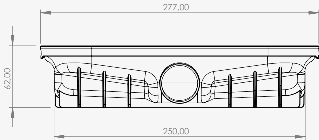
TRYPHON RIDOTTO: Uscita DN/DE 40 mm
