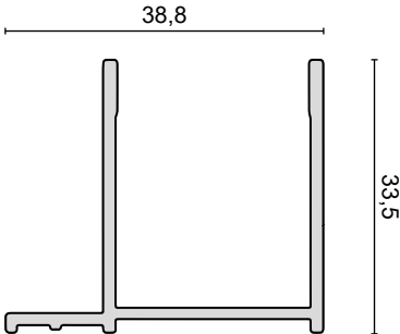
PROFILO A MURO - WALL PROFILE WANDPROFIL- PROFIL DE MUR
