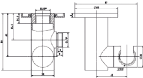
LSRMT 01B
