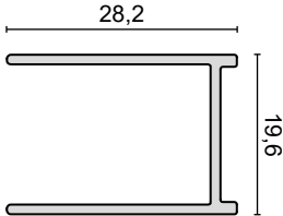
PROFILO A MURO WALL PROFILE - WANDPROFIL - PROFIL DE MUR
