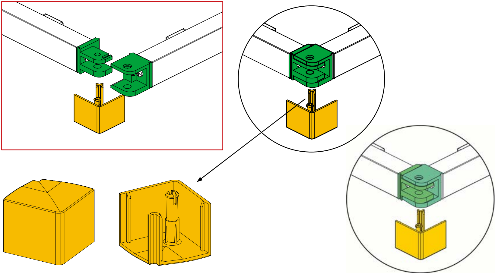
UNIRE I DUE PROFILI ORIZZONTALI COME INDICATO IN DISEGNO E POI CHIUDERE IL TUTTO CON IL CORNER.
