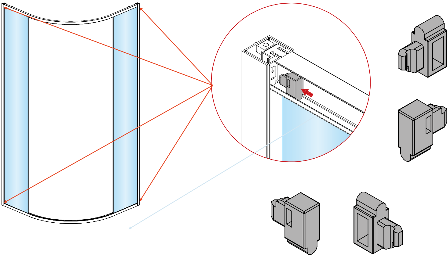
INSERIRE IL PEZZO INDICATO NEL PROFILO VERTICALE IN MODO TALE DA BLOCCARE IL MONTAGGIO TRA IL PROFILO ORIZZONTALE E QUELLO VERTICALE.
