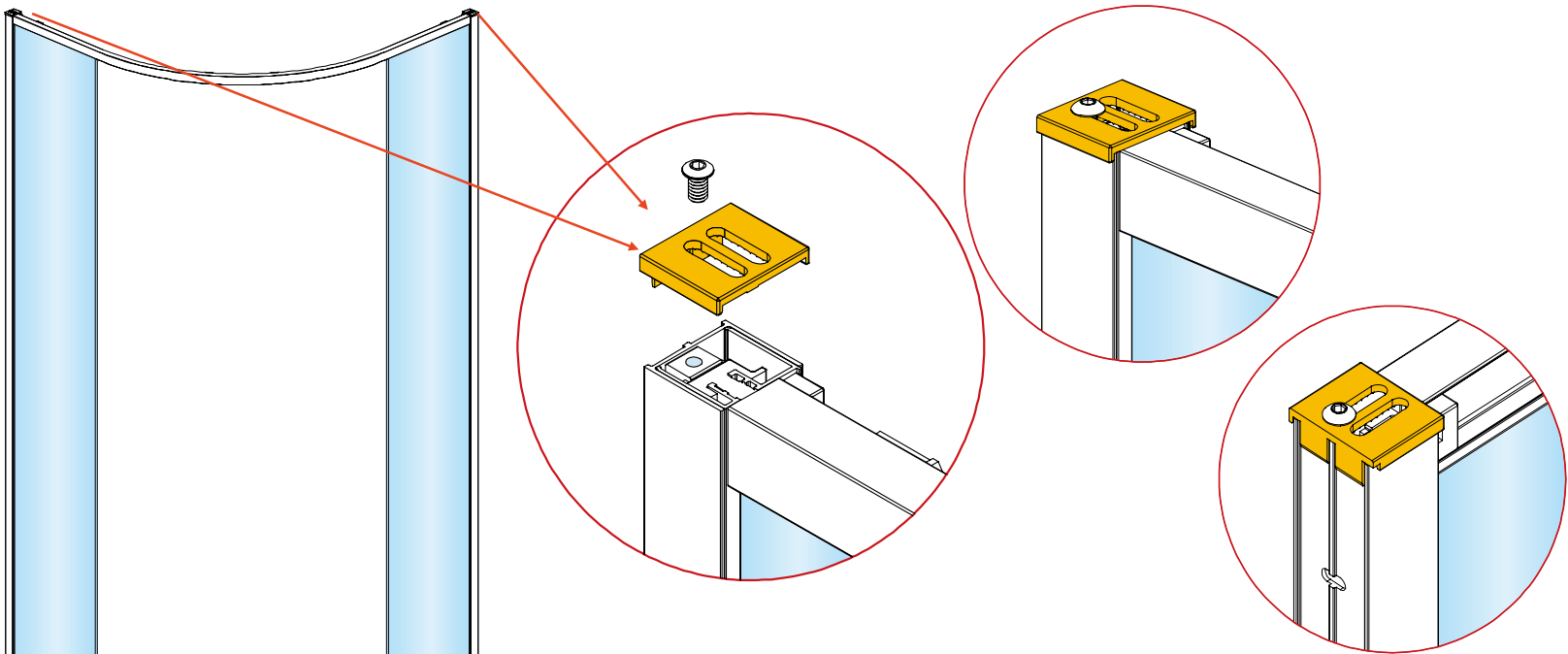
REGOLARE L'ESTENSIONE DEL PROFILO A MURO TRAMITE IL COPRIPROFILO.
