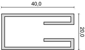
PROFILO A MURO WALL PROFILE - WANDPROFIL - PROFIL DE MUR
