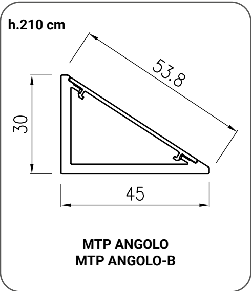
Profilo angolare per fissaggio laterale. Corner profile for lateral fixing. Winkelprofil zur seitlichen Befestigung. Profilé angulaire pour fixation latérale.
